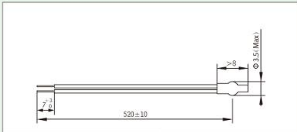
PTC single sensor mini
