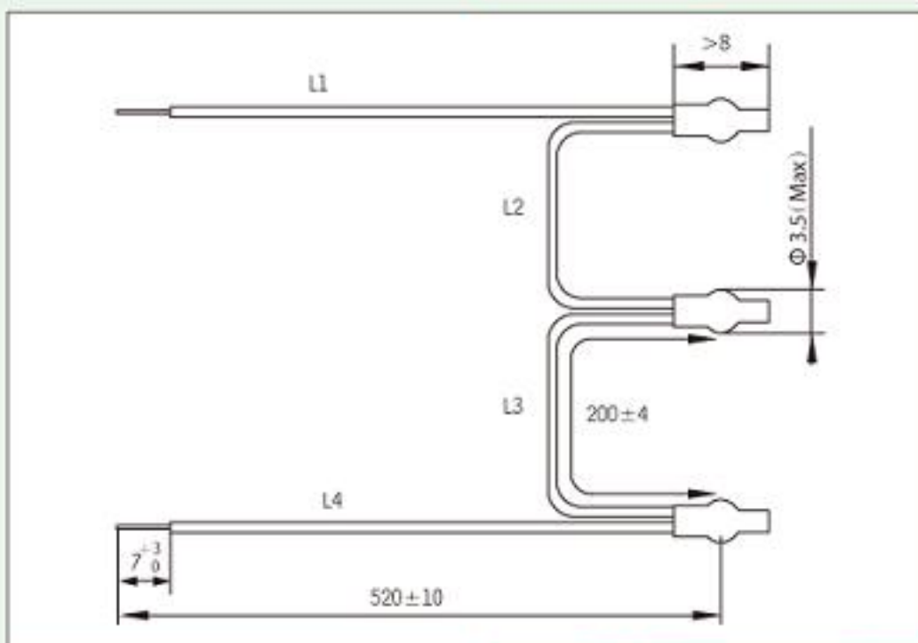
PTC triple sensor mini
